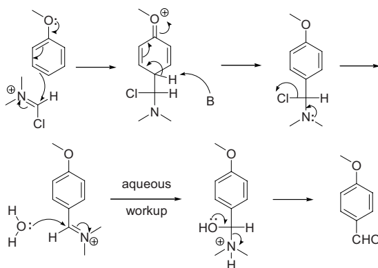
Vilsmeier–Haack reagent
